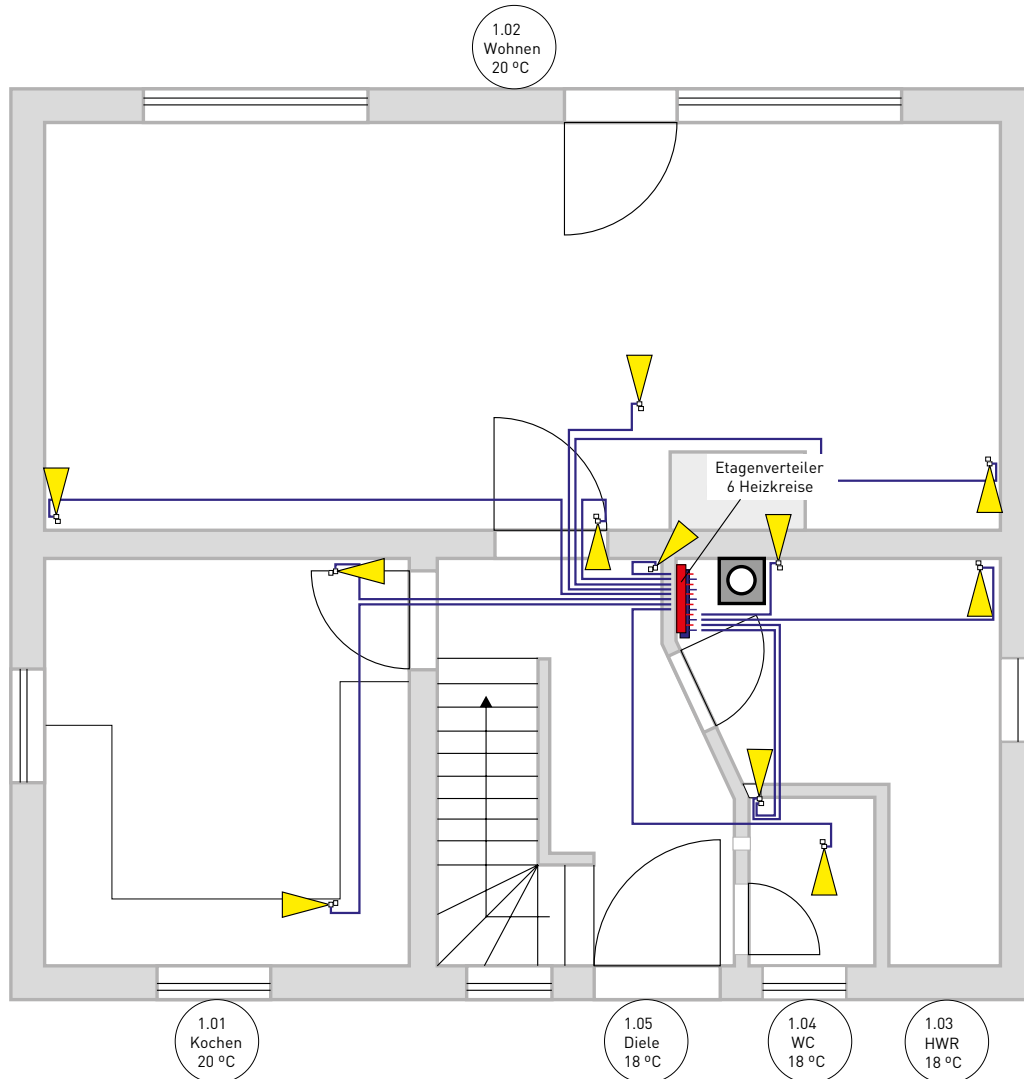
Strangschema
